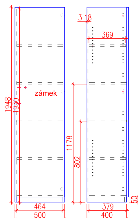
AT 555 1KS Korpusy DTD-L 112 PE ŠEDÁ/ABS 2mm Dvířka H1277 akacie/abs 2mm Úychtka kovová rozteč 160mm barva černá broušená Nk závěsy Blum s integrovaným tlumením Zámek Rektifikační nožka korrekt 50mm
