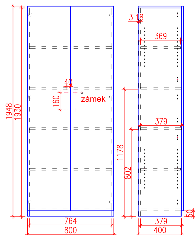
AT 555 Š 2KS 1x dveře levé 1xdveře pravé Korpusy DTD-L 112 PE ŠEDÁ/ABS 2mm Dvířka H1277 akacie/abs 2mm Úychtka kovová rozteč 160mm barva černá broušená Nk závěsy Blum s integrovaným tlumením Šatní výsuv Zámek rozvorový Rektifikační nožka korrekt 50mm
