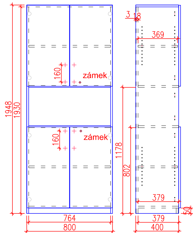
AT 582.2 2KS Korpusy DTD-L 112 PE ŠEDÁ/ABS 2mm Dvířka H1277 akacie/abs 2mm Úychtka kovová rozteč 160mm barva černá broušená Nk závěsy Blum s integrovaným tlumením Zámek Rektifikační nožka korrekt 50mm
