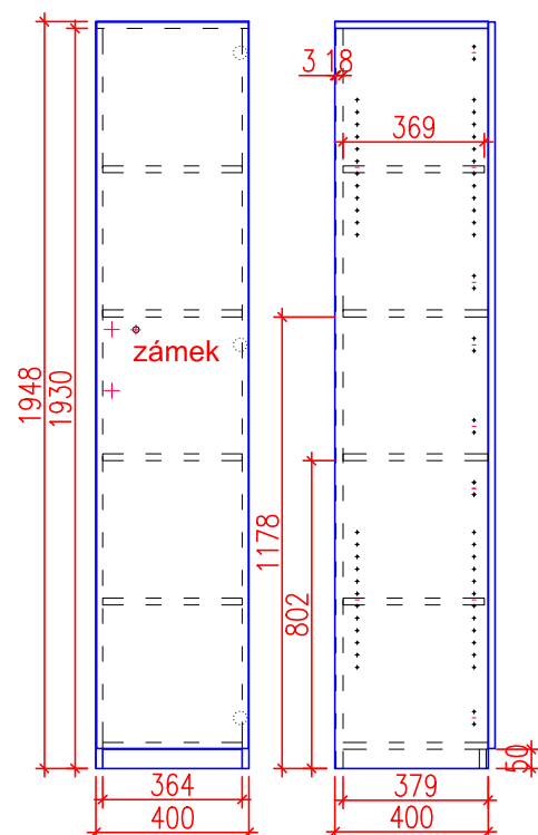
AT 545 1KS Korpusy DTD-L 112 PE ŠEDÁ/ABS 2mm Dvířka H1277 akacie/abs 2mm Úychtka kovová rozteč 160mm barva černá broušená Nk závěsy Blum s integrovaným tlumením Zámek Rektifikační nožka korrekt 50mm
