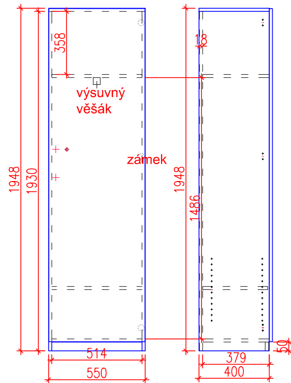
AT 555 Š 2KS 1x dveře levé 1xdveře pravé Korpusy DTD-L 112 PE ŠEDÁ/ABS 2mm Dvířka H1277 akacie/abs 2mm Úychtka kovová rozteč 160mm barva černá broušená Nk závěsy Blum s integrovaným tlumením Šatní výsuv Zámek rozvorový Rektifikační nožka korrekt 50mm
