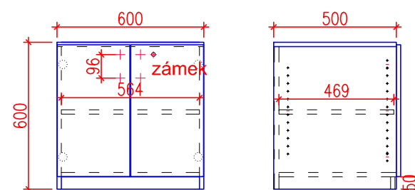
AT 555 1KS Korpusy DTD-L 112 PE ŠEDÁ/ABS 2mm Dvířka H1277 akacie/abs 2mm Úychtka kovová rozteč 160mm barva černá broušená Nk závěsy Blum s integrovaným tlumením Zámek Rektifikační nožka korrekt 50mm
